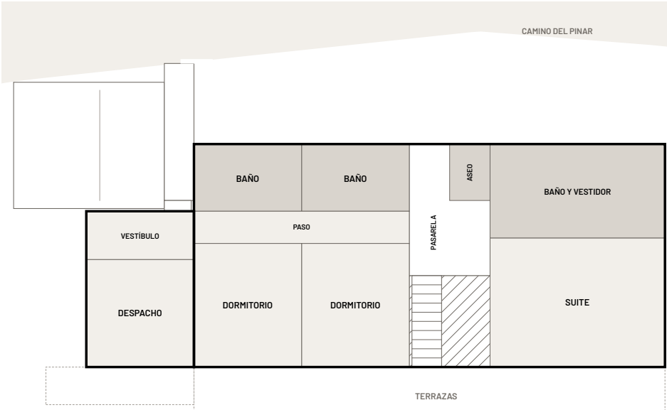
SUITE Y DOS DORMITORIOS CON BAÑO · VESTÍBULO Y DESPACHO SOBRE EL CINE
