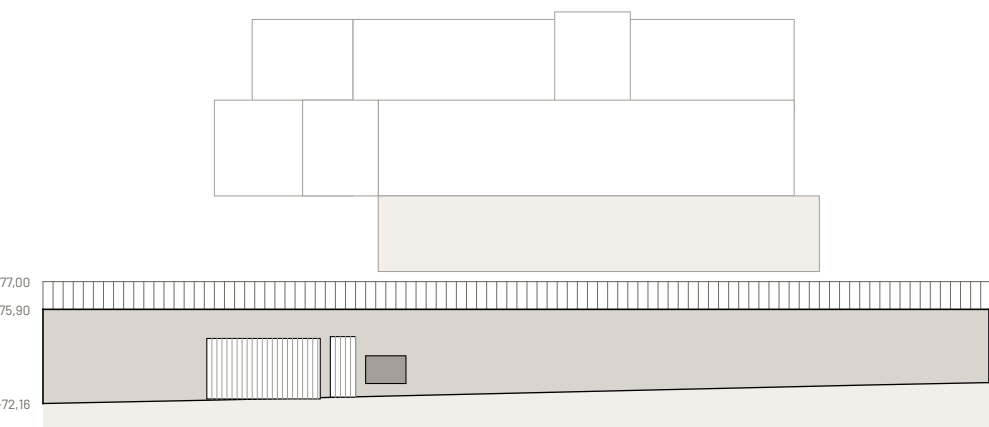
ALZADO AL CAMINO DEL PINAR 1:300
